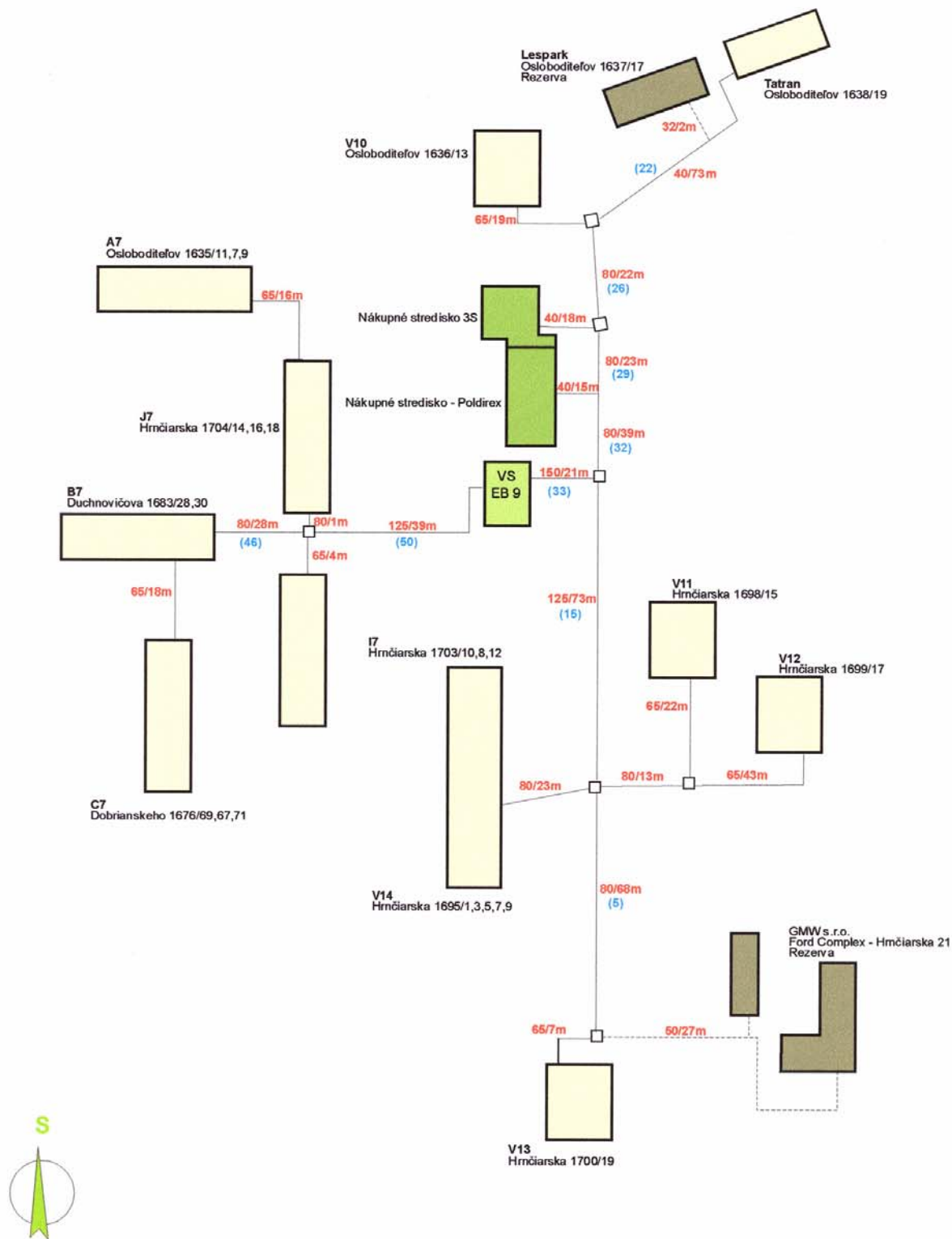
SITUAČNÁ SCHÉMA SEKUNDÁRNYCH ROZVODOV - VS EB 9 Hrnčiarska
